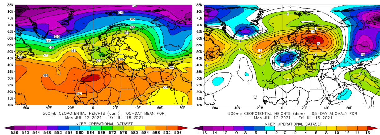
Abbildung 7: Höhe der gemittelten 500 hPa-Geopotentialfläche in gpdm und deren Abweichung vom langjährigen Mittelwert des Zeitraum 1981 bis 2010. Mittelungszeitraum: 5 Tage (12. bis 16.07.2021; Quelle: https://psl.noaa.gov/data/histdata ).
