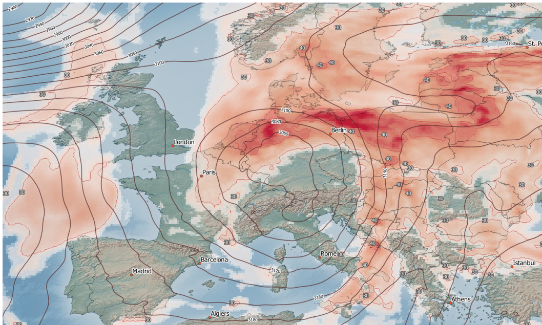
Abbildung 5: Analyse der 700 hPa-Geopotentialfläche (dünne dunkelgraue Linien) sowie die Menge des in der der Atmosphäre verfügbaren ausfällbaren Wassers in mm (rote Farbflecken und rote Linien) vom 14. Juli 2021, 12UTC. (Modelldaten: GEM).
